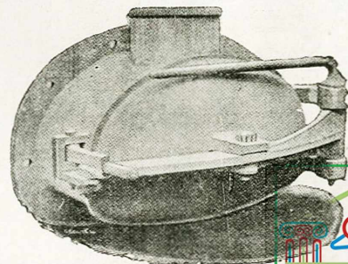
Têtes de cornues sans lut
