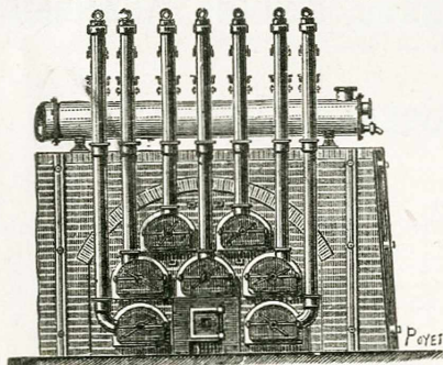
Ensemble d'un four à 7 cornues
