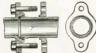
Têtes de cornues sans lut
